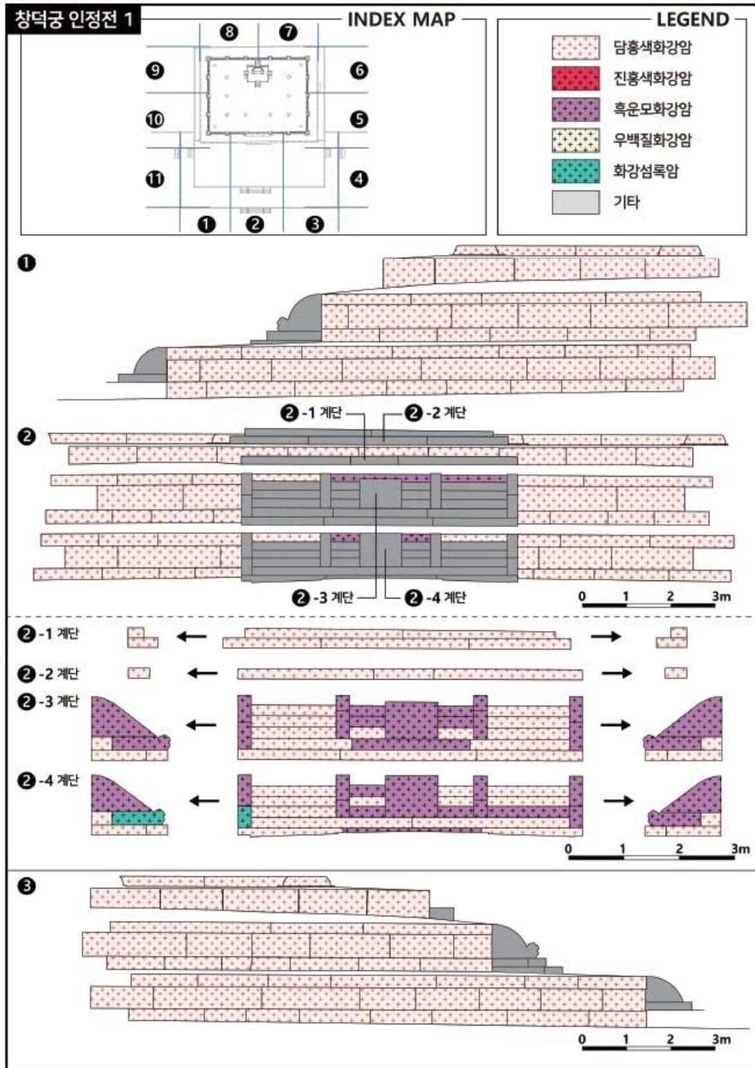
< 창덕궁 인정전 암석도면(일부) >
